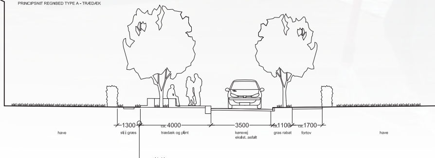
PRINCIPSNIT REGNBED TYPE A - TRÆDÆK
